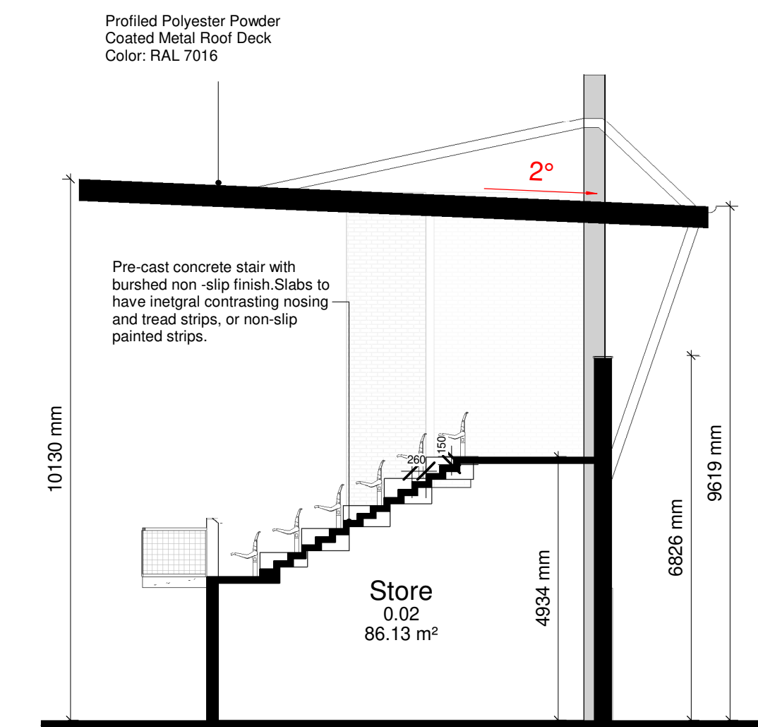
1. Section 1 1 : 100
